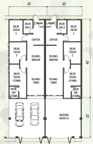
Pelan Lantai
